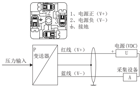
电流输出接线图8-4(两线制)
