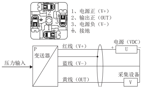
电压输出接线图8-5(三线制)
